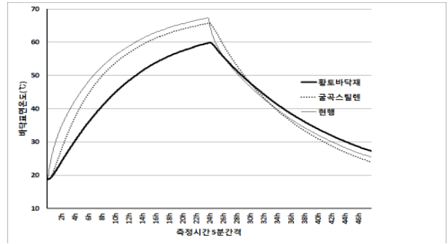
그림 7. 습식구조 60°C 난방 및 냉각시 바닥표면온도 변화
