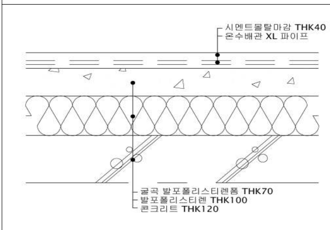
굵은 스틸렌폼 온수온돌 구조
