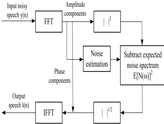
그림 2. 기존의 스펙트럼 차감법의 블록도 Fig. 2 Block diagram of conventional spectrum subtraction
