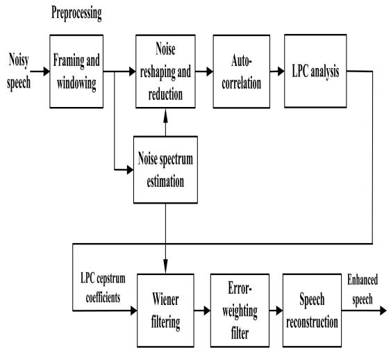
그림 3. 제안하는 위너 필터 알고리즘 Fig. 3 Proposed wiener filter algorithm
