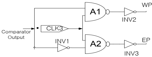
그림 5. PTDC 회로도 Fig. 5 PTDC circuit diagram
