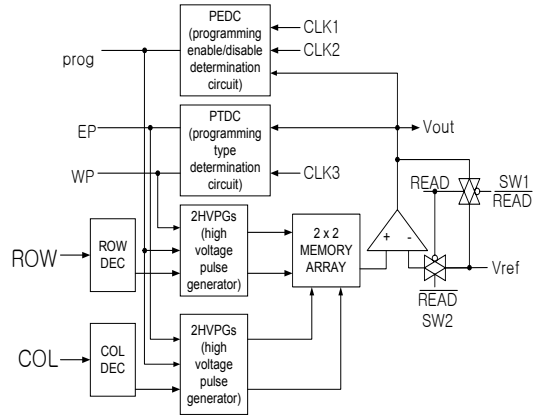
그림 2. 2x2 아날로그 메모리의 블록도 Fig. 2 A 2x2 analog memory block diagram
