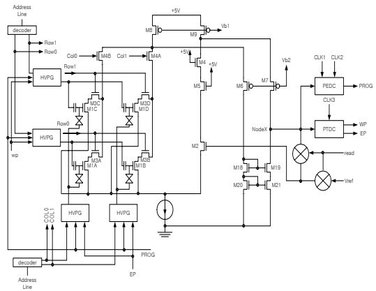
그림 3. 2x2 아날로그 메모리 회로도 Fig. 3 A 2x2 Analog memory circuit diagram
