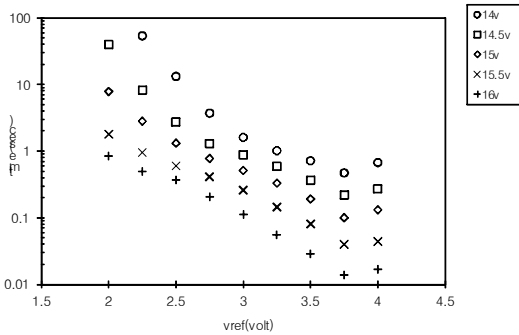
그림 10. 프로그래밍 펄스의 크기와 시간간의 특성 곡선 Fig. 10 Elapsed time vs. programming pulse magnitude
