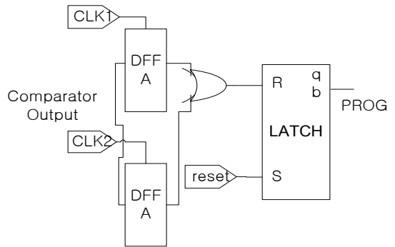
그림 4. PEDC 회로도 Fig. 4 PEDC circuit diagram
