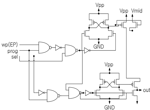
그림 6. HVPG 회로도 Fig. 6 HVPG circuit diagram
