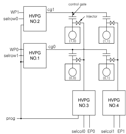
그림 7. 단순화된 2x2 어레이 블록도 Fig. 7 A simplified block diagram of 2x2 array
