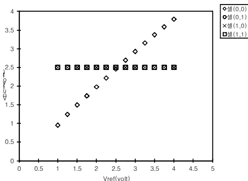
그림 11. 특정 셀 (0,0) 프로그래밍 시의 간섭효과 Fig. 11 Disturbance effect as a cell (0,0) being selected for programming.
