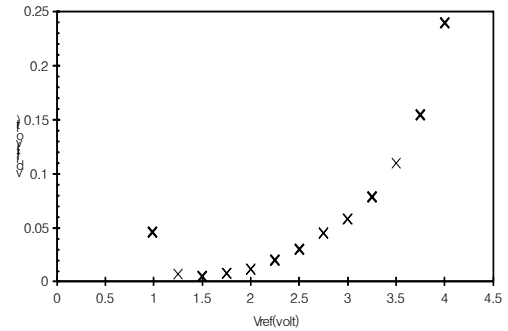
그림 9. 프로그래밍 전과 후의 전압 오차 Fig. 9 Magnitude of mismatch between stored and reference voltage
