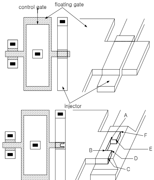
그림 1. type 1과 type 2의 평면도와 입체도 (a) type 1 (b) type 2
