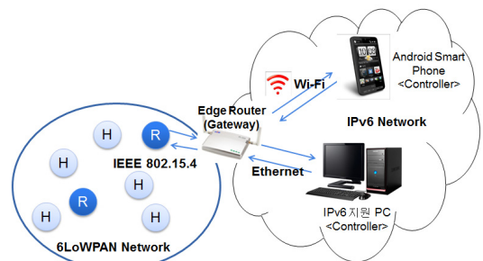
그림 2. IP-USN 시스템 아키텍처 Fig. 2. IP-USN system architecture
