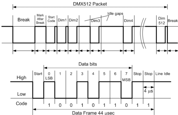
그림 4. DMX512 프로토콜 프레임 구조 Fig. 4. Frame structure of DMX512 protocol
