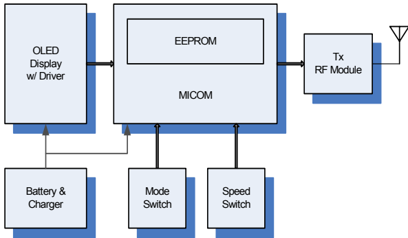
그림 7. LED 주제어기 리모콘 Fig. 7. Block diagram of remote controller
