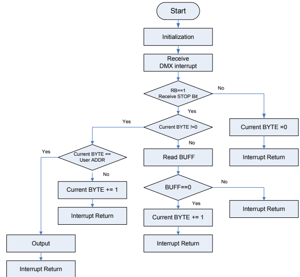
그림 8. 데이터 수신 알고리즘 Fig. 8. Data receiving algorithm
