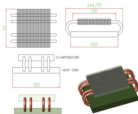
그림 2. 고출력 LED 방열용 히트 파이프 설계 Fig. 2. Heat-pipe design for High-powered LED
