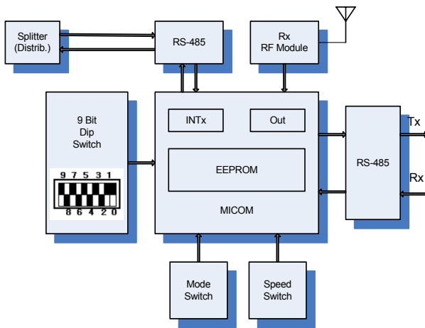
그림 6. 주제어기 블록도 Fig. 6 Block diagram of main controller
