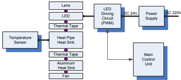
그림 1. 고출력 LED 투광등의 방열 구조 Fig. 1. High-powered LED Heat-sink structure
