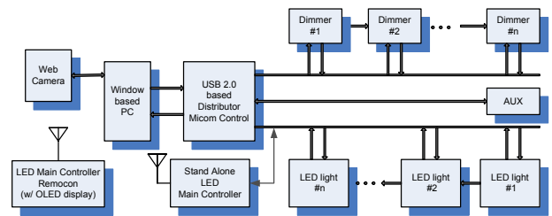
그림 5. LED 투광기 시스템의 전체 네트워크 구성도 Fig. 5. Network diagram for LEDs using DMX512
