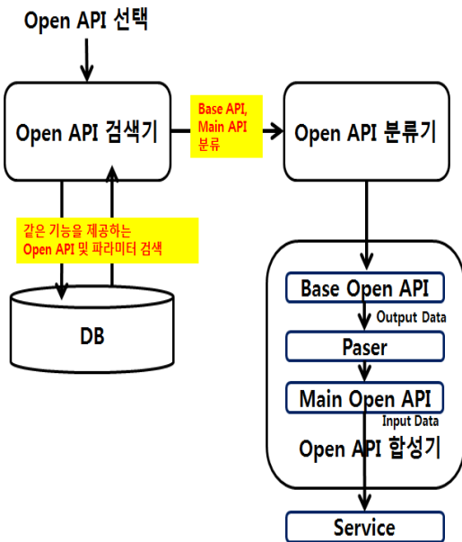
그림 7. Open API 분류기 및 합성기 구조 Fig. 7. Structure of Open API Classifier and Composer
