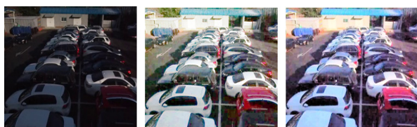
(a) 입력 영상 (b) 독립 채널 변환 (c) 밝기유지 변환 (a) Reference image (b) Channel compensation (c) Luminance compensation 그림 1. 컬러 히스토그램 평활화 결과 Fig. 1. Color histogram equalization
