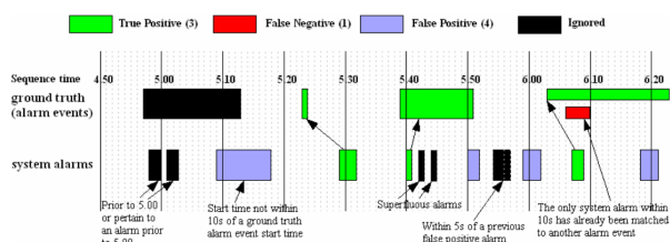
그림 9. iLIDS의 결과 검출 방식 Fig. 9. Result calculation method of iLIDS
