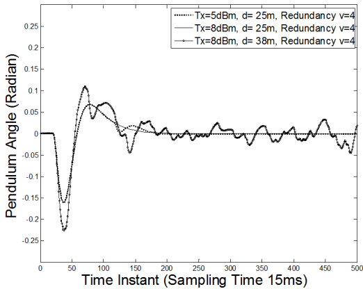
그림 11. 중복 전송 슬롯 4개 사용시 역진자 시스템 응답 Fig 11. System response of Inverted Pendulum with 4 Redundancy
