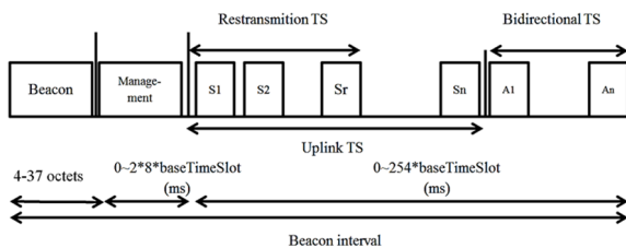
그림 2. LL MAC 슈퍼 프레임 구조 Fig. 2. Structure of LL MAC Super-frame
