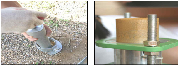
그림 1. 공시체 제작
