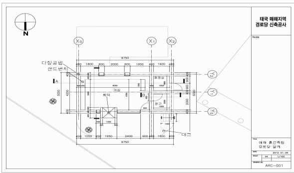
그림 5. 평면도
