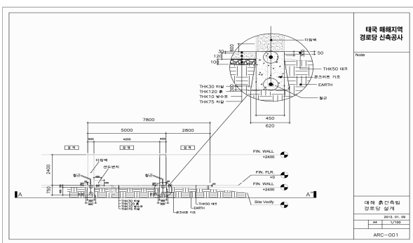
그림 7. 단면도
