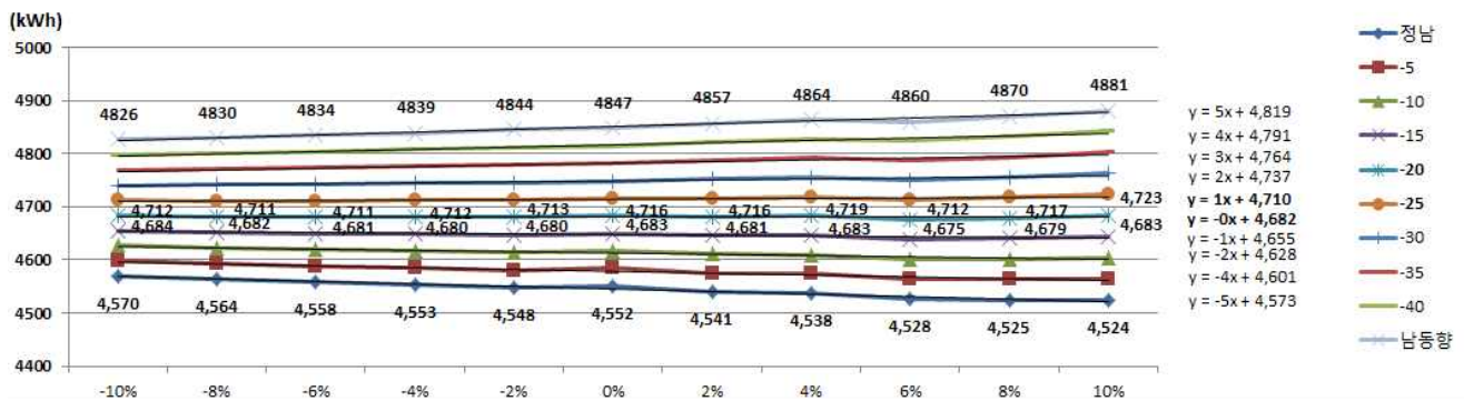
그림 3. 임대형(46㎡)의 정남에서 남동향 사이 9개 구간(5°간격)의 연간 냉난방 에너지요구량(kWh) 그래프
