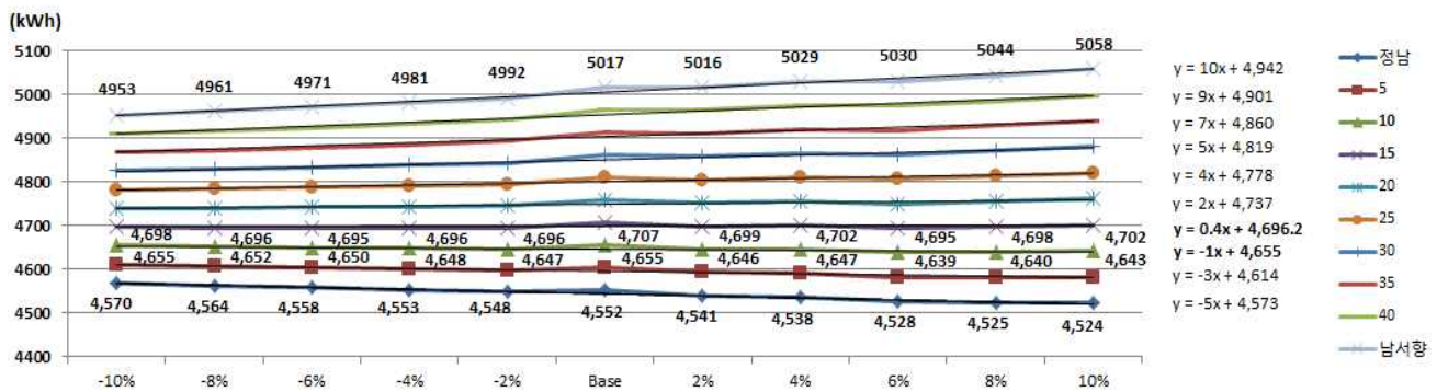
그림 2. 임대형(46㎡)의 정남에서 남서향 사이 9개 구간(5°간격)의 연간 냉난방 에너지요구량(kWh) 그래프
