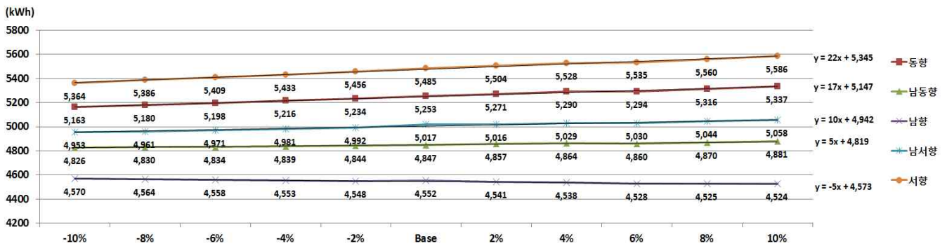
그림 1. 임대형(46㎡)의 향별 창면적비 변화에 따른 연간 냉난방 에너지요구량(kWh) 그래프
