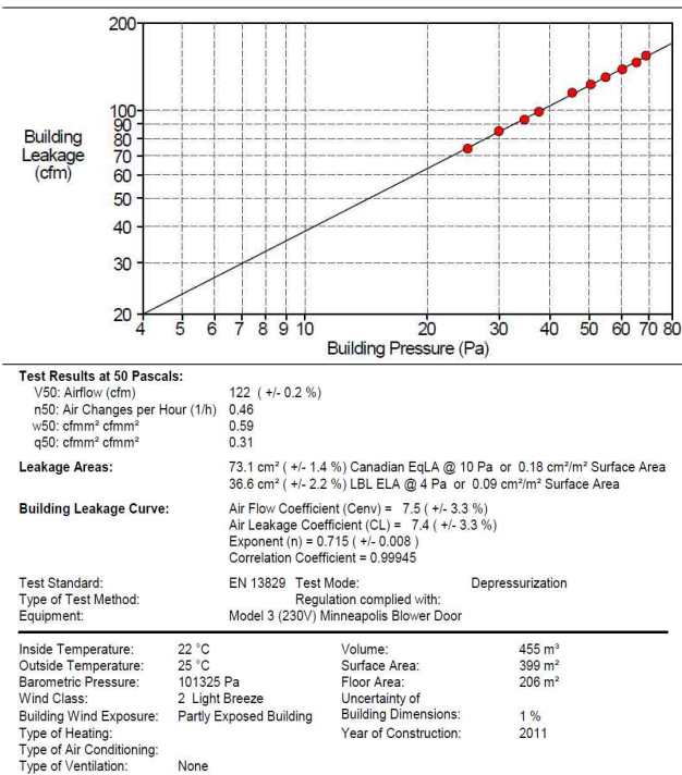
그림 3-1. ALT-1 Test Results at 50 Pascals(기밀성능치)
