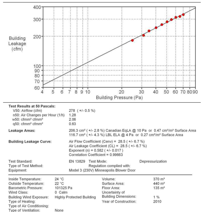
그림 3-3. ALT-2 Test Results at 50 Pascals(기밀성능치)
