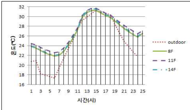
그림 7. 발코니 온도분포(Case 3)
