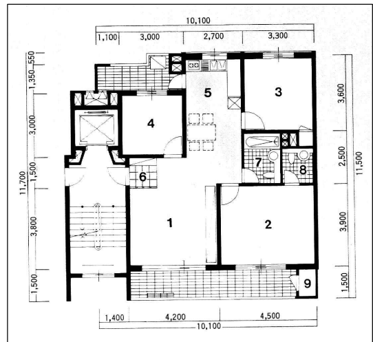
그림 1. 대상모델 평면
