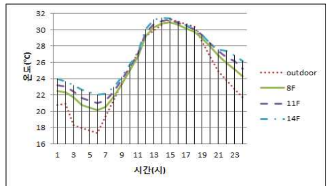
그림 11. 발코니 온도분포(Case 4)
