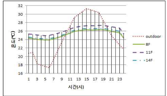
그림 3. 실내 온도분포(Case 1)
