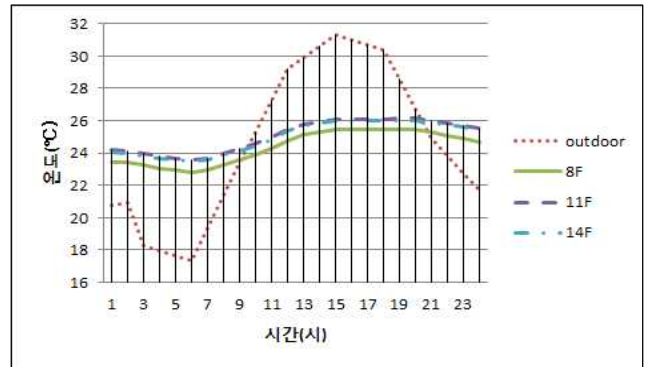
그림 10. 실내 온도분포(Case 4)
