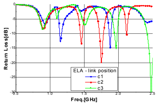
<그림 4> 상단 연장 루프 연결점(a)별 반사손실(b) <Fig. 4> Return losses(b) vs. connection points of upside extended loop(a)
