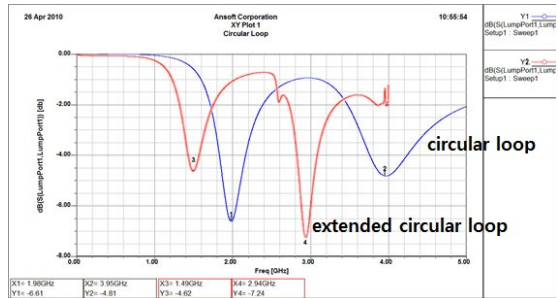
<그림 2> 그림 1 루프안테나의 공진특성 <Fig. 2> Resonances of Fig. 1 loop antennas
