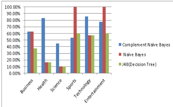
그림 9. 구글 뉴스 메타 태그의 분류 알고리즘 정확도 Fig. 9. Accuracy of the classification algorithm(Google news meta tags and Google News meta tags text)
