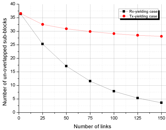
그림 5. Tx/Rx-block 내 중첩이 되지 않은 sub-block 수 ( N_{SUB} = 40, N_T \times N_F = 4 \times 15 ) Fig. 5. The number of un-overlapped sub-blocks in Tx/Rx-block ( N_{SUB} = 40, N_T \times N_F = 4 \times 15 )
