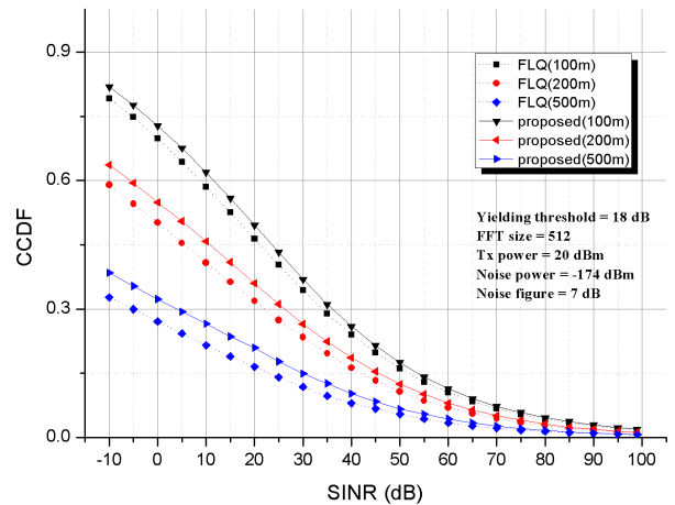
그림 10. 스케줄링된 링크들에 대한 SIR CCDF 비교 (Threshold = 18 dB, N = 105) Fig. 10. Comparison of SIR CCDF as the number of scheduled links changes (Threshold = 18 dB, N = 105)
