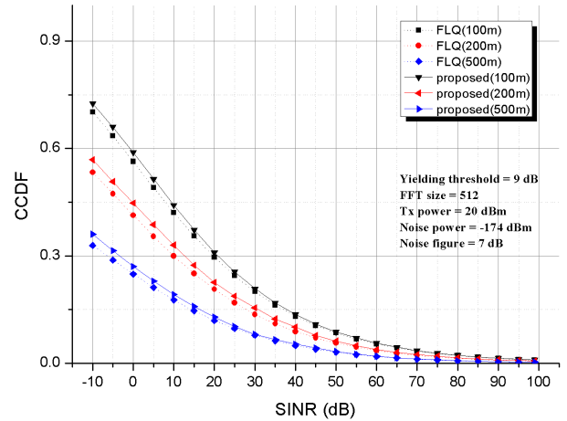
그림 9. 스케줄링된 링크들에 대한 SIR CCDF 비교 (Threshold = 9 dB, N = 105) Fig. 9. Comparison of SIR CCDF as the number of scheduled links changes (Threshold = 9 dB, N = 105)
