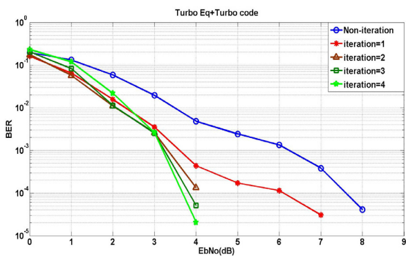
그림 9. BER 성능 Fig. 9. BER Performance
