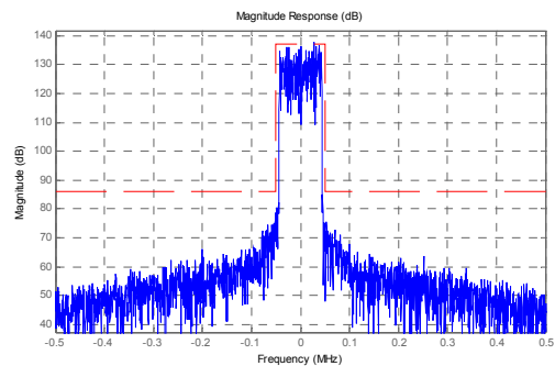
그림 13. 100kHz 초단파 데이터 시스템에서 25배 업샘플링 인터플레이션 필터의 크기응답 Fig. 13. Magnitude response of interpolation filter with upsampling by a factor of 25 for the 100kHz VHF data system
