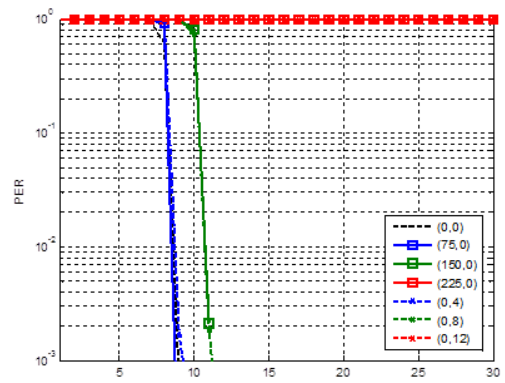
그림 7. AWGN에서 100kHz 대역 시스템의 PER 특성 (주파수오차(Hz), 시간오차(samples)) Fig. 7. PER of 100kHz system under AWGN with frequency offset and timing offset
