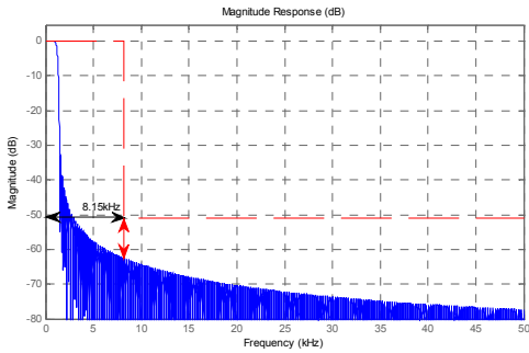
그림 10. 100kHz 초단파 데이터 시스템에서 865탭 펄스형필터의 크기 응답 (12심볼주기) Fig. 10. Magnitude response of 865-tap pulse shaping filter for the 100kHz VHF data system (12-symbol interval)
