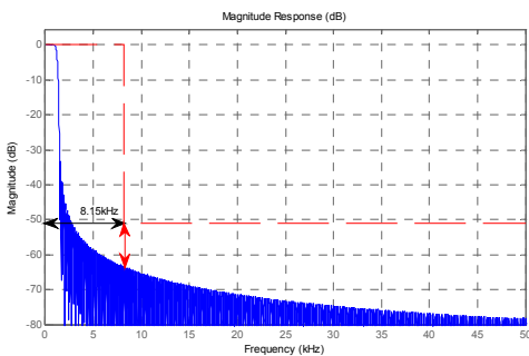
그림 11. 100kHz 초단파 데이터 시스템에서 937탭 펄스형필터의 크기 응답 (13심볼주기) Fig. 11. Magnitude response of 937-tap pulse shaping filter for the 100kHz VHF data system (13-symbol interval)
