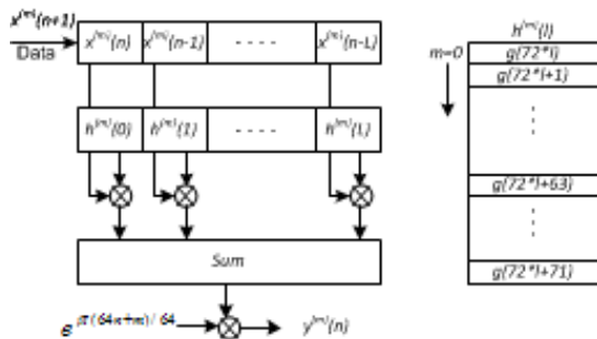
그림 6. Polyphase 필터 बैं크의 구현방식 Fig. 6. Implementation of Polyphase Filter bank
