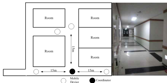
그림 5. 실험 수행 환경 Fig 5. The Test Environment
