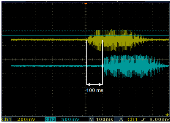
그림 6. 음성 전송 지연 측정 그래프 Fig 6. The Graph of Voice Packet Delay Measurement
