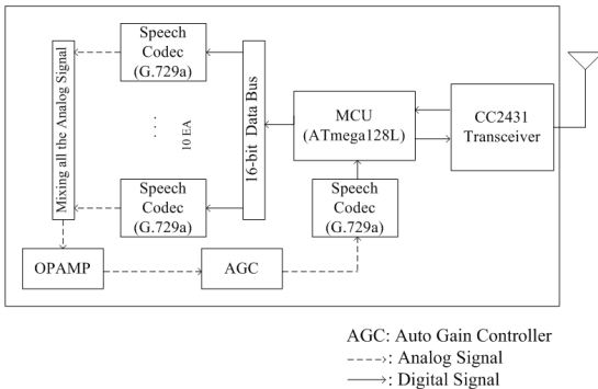
그림 3. 센서 네트워크 기반 다수 사용자간 Full-Duplex 음성 통신을 위한 Coordinator의 Block Diagram Fig 3. The Block Diagram of Coordinator for Full-Duplex Multi-User Voice Communication Systems Based on Sensor Network
