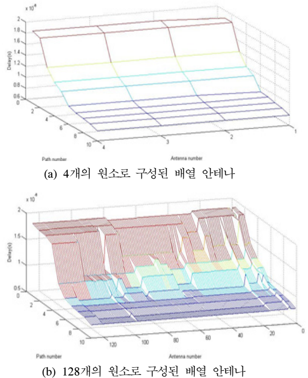
그림 2. 안테나-지연 산란 함수 Fig 2. Antenna-delay scattering function
