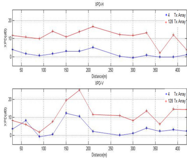
(위) 송신 편파가 수평 편파인 경우의 교차 편파 식별도 (아래) 송신 편파가 수직 편파인 경우의 교차 편파 식별도 그림 5. 교차 편파 식별도 비교 Fig 5. XPD comparison
