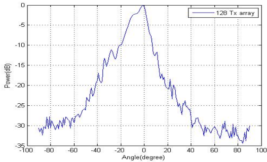
(b) 128 Tx Array의 PAS
