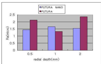
(b) 표면조도
