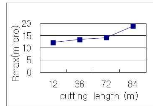
(b) 표면조도
