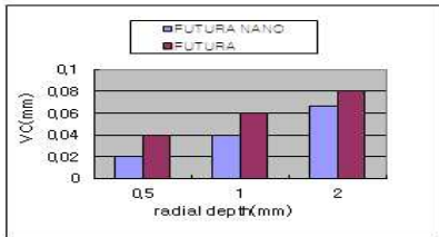
(a) 여유면마모량
