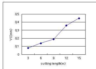
(a) 여유면마모량
