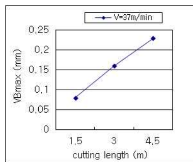
Fig.3. V=37m/min에서 여유면 마모량(uncoating).
