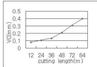
(a) 여유면마모량
