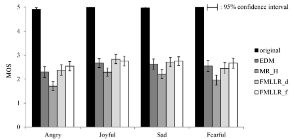
그림 4. 여성 음성의 주관적 듣기 평가 결과. Fig. 4. Result of subjective listening test for female voice.
