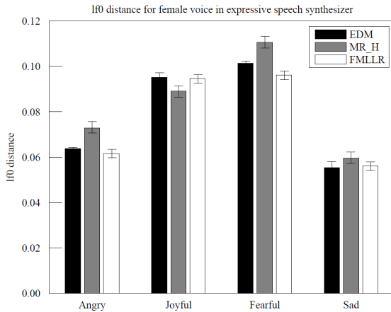
그림 2. 여성 음성 평균 lf0 distance. Fig. 2. Average lf0 distance for female voice.
