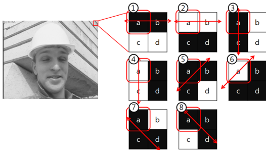
그림 9. 윤곽선의 패턴 고려를 위한 2*2 블록의 8가지 패턴
