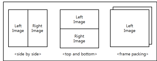
[Fig. 1] Stereo Video Data Forat
