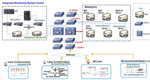
(그림 8) 통합 모니터링 시스템 구성도
