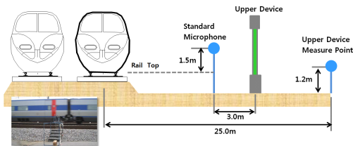
(그림 2) 방음벽 상단장치 성능평가 구성도
