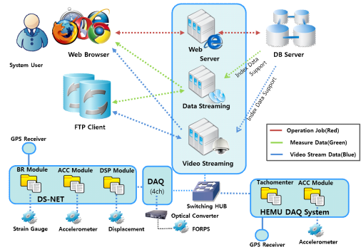
(그림 4) 궤도 모니터링 통합계획
