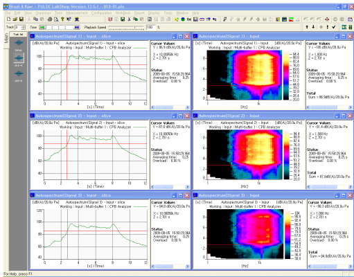
(a) 시간-음압레벨 선도 (b) 주파수-음압레벨 선도 (그림 5) 상용프로그램을 이용한 측정위치별 분석결과
