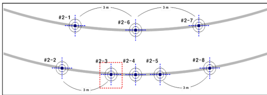
(그림 3) 궤도부(원곡선구간) 센서배치 구성도
