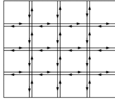
그림 6. Manhattan 모델 [14]
