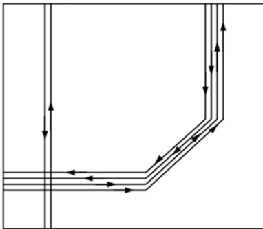
그림 5. Freeway 모델 [14]
