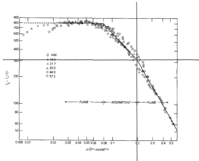
[도표] 화염 높이에 따른 온도 변화 (프로판 화재 실험에서 플럼과 중간영역 부근의 온도는 300°C를 조금 넘고 있다.)
