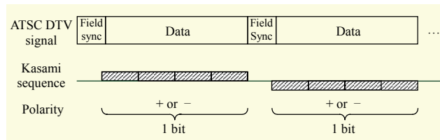
Fig. 3. 40-bps mode.
