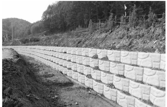
하천 법면 보호용(시공사진)
