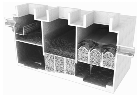
초기우수처리시설(EGS-System)
