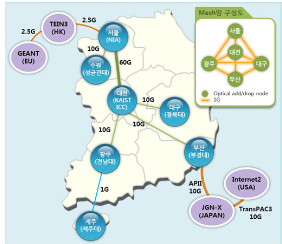
그림 6. KOREN 토폴로지 구성도 Fig. 6. KOREN Topology Map
