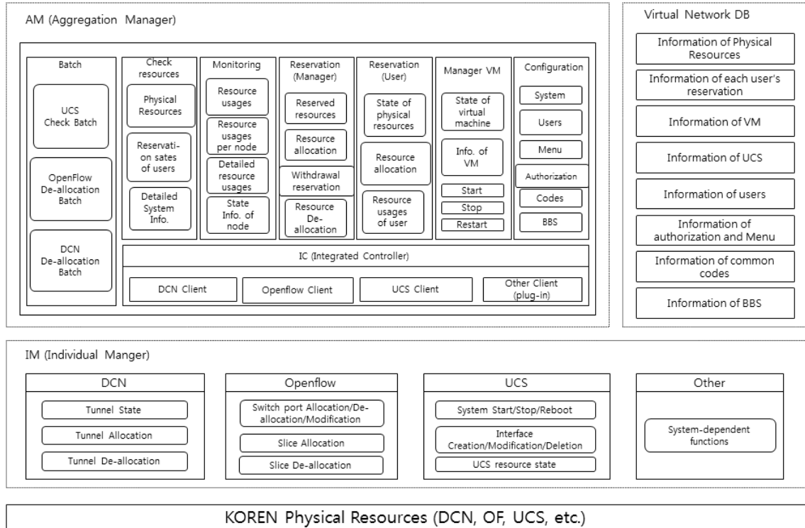
그림 3. 가상네트워크 통합제어 프레임워크 Fig. 3. Framework of virtual network integrated management system
