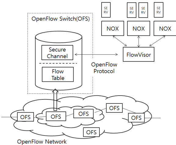
그림 2. OpenFlow스위치 및 네트워크 구성도 Fig. 2. Architecture of OpenFlow switch and network
