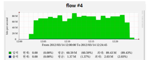
그림 11. 시나리오 B 실험결과 Fig. 11. Test result of scenario B
