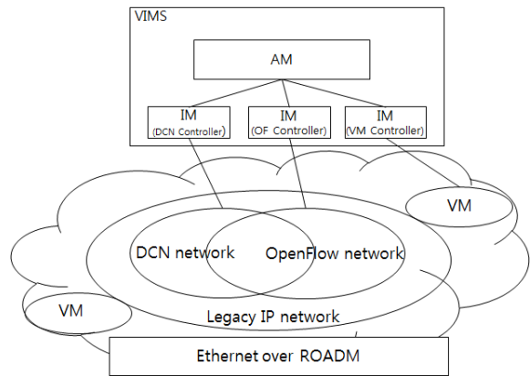
그림 7. 가상네트워크 환경 구성도 Fig. 7. Diagram of virtual network environment on KOREN
