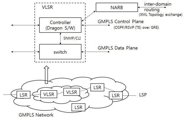
그림 1. DCN의 VLSR 구성도 Fig. 1. Architecture of DCN VLSR
