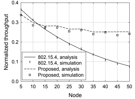
그림 6. Saturated 트래픽 환경에서 센서 노드 수의 변화에 따른 normalized throughput의 차이
