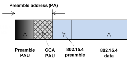
그림 1. 제안 기법의 패킷 전송 기본 구조 Fig. 1. Preamble construction and integration with an 802.15.4 packet
