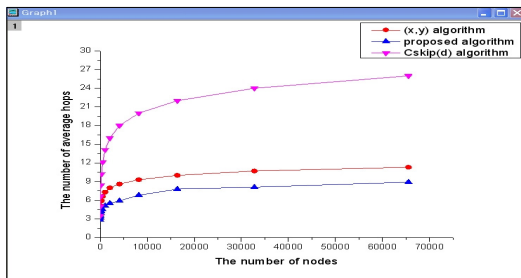
그림 14. (8, 4, 4) 좌표 총 65,536개 노드 Fig. 14. (8, 4, 4) coordinate the total node 65,536
