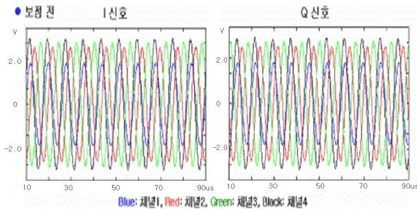
그림 12 수신 출력신호의 크기와 위상 보정 전 Fig. 12 Before calibration of amplitude and phase in output signal
