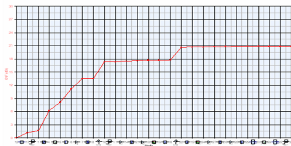
그림 4 수신 잡음지수 특성 Fig. 4 Noise figure Characteristics
