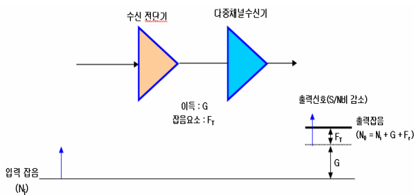
그림 2 전체 수신 잡음 지수의 개념도 Fig. 2 Concept of total noise figure
