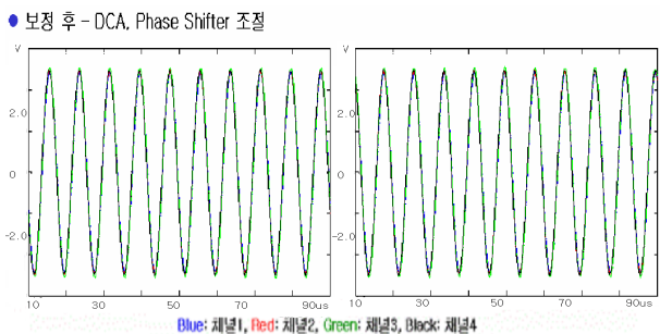
그림 13 수신 출력신호의 크기와 위상 보정 후 Fig. 13 After calibration amplitude and phase in output signal
