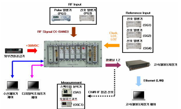
그림 9 다채널 수신기 측정 구성도 Fig. 9 Test system of multi channel receiver
