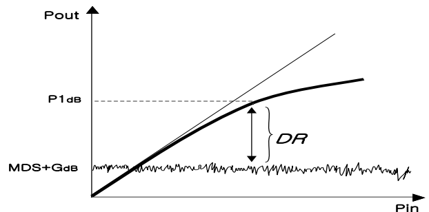
그림 7 수신기 입력 동특성 Fig. 7 Input dynamic range in receiver
