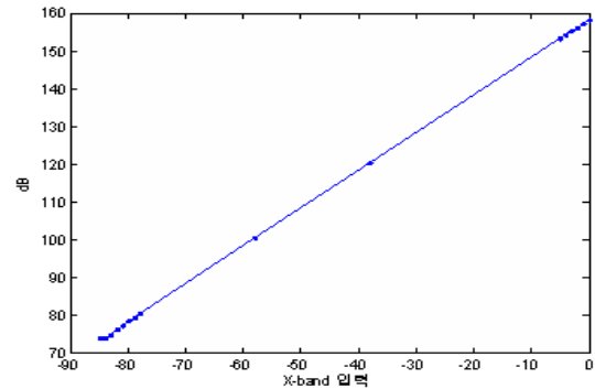
그림 14 안테나 S11 측정결과 Fig. 14 Result of antenna S11 measurement
