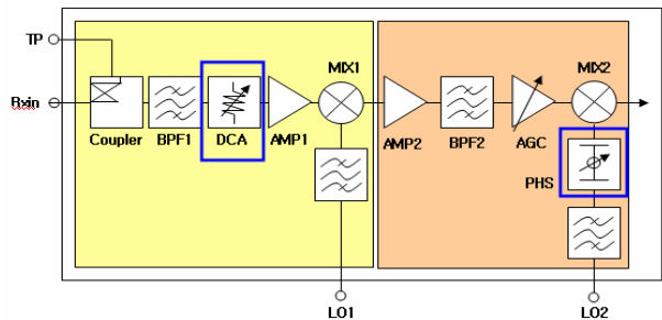
그림 6 DCA와 위상변위기를 적용한 수신시스템 Fig. 6 Receiver system using DCA & Phase shift
