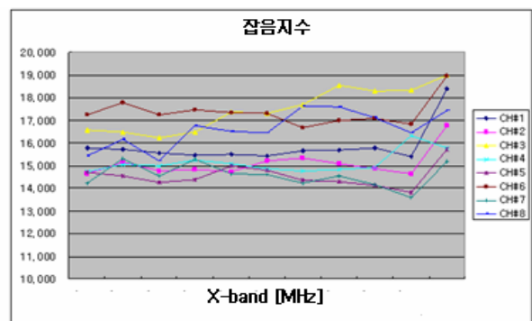
그림 10 수신기(채널) 별 잡음 지수 Fig. 10 Noise Figure at each channel
