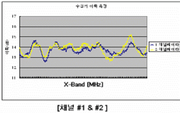
그림 11 수신채널 #1 및 #2의 수신이득 Fig. 11 Gain at channel #1 and #2
