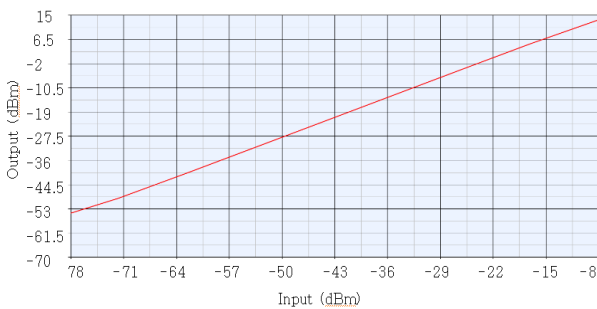
그림 8 80dB에 대한 수신 동특성 Fig. 8 The receiver dynamic range for 80dB
