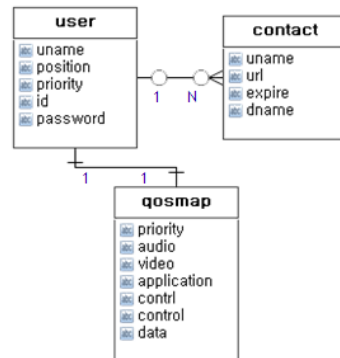
그림 2. 가입자 정보 관리 테이블 Fig. 2 Table of subscriber information
