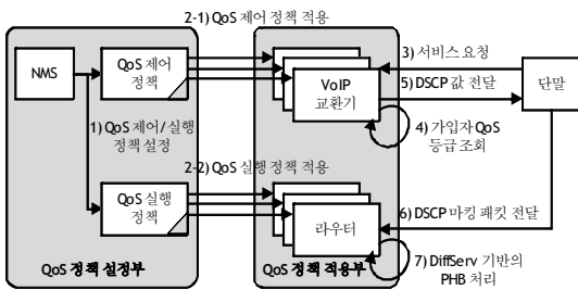
그림 1. 전술통신환경에서의 Dynamic QoS 구조 Fig. 1 Dynamic QoS in tactical communication
