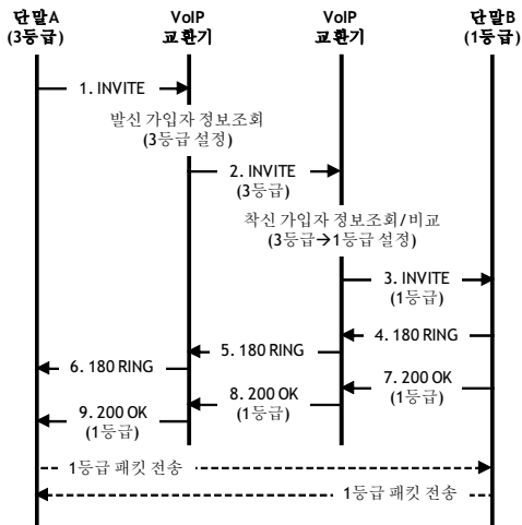
그림 6. 호 처리 흐름도(타 교환기) Fig. 6 Call Flow(between two VoIP System)
