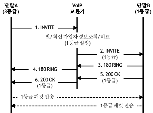
그림 5. 호 처리 흐름도(동일 교환기) Fig. 5 Call Flow(in a VoIP system)
