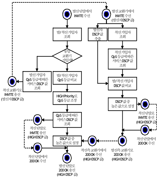
그림 3. 가입자 QoS 등급 조회 알고리즘 Fig. 3 DSCP decision algorithm
