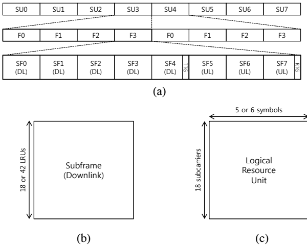
그림 2. 프레임 구조 Fig. 2. Frame Structure
