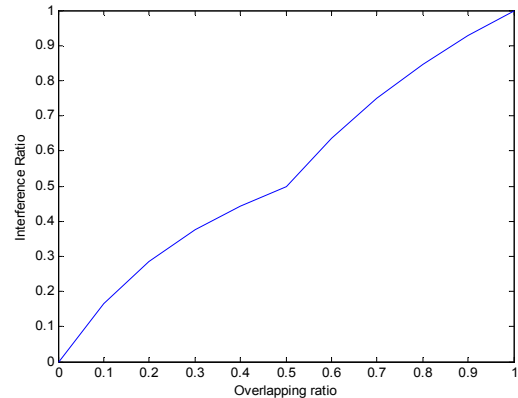
그림 5. 실효 간섭 비율 Fig. 5. Effective Interference Ratio
