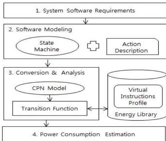
그림 1. 상태 기반의 소모전력 분석 절차 Fig. 1. State-based software power analysis process
