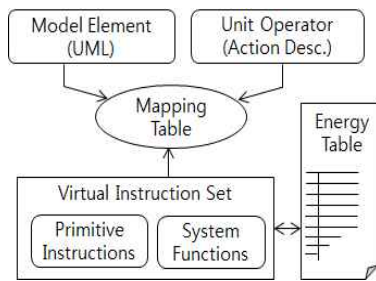
그림 2. 에너지 라이브러리의 구조 Fig. 2. The structure of energy library
