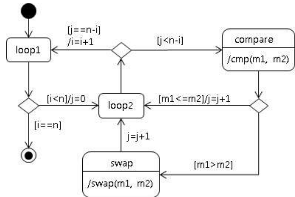
(a) Bubble Sort 상태기계 다이어그램
