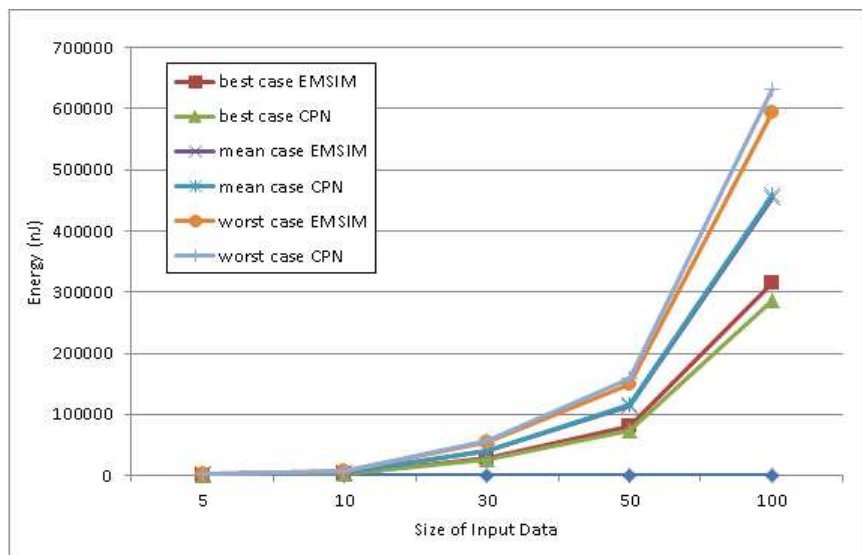
그림 9. 버블정렬에 대한 소모전력 측정 값 Fig. 9. Energy consumption graph for bubble sort
