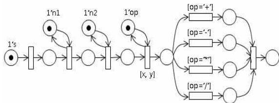
그림 5. 사칙연산자의 CPN 모델 Fig. 5. CPN model of arithmetic operators
