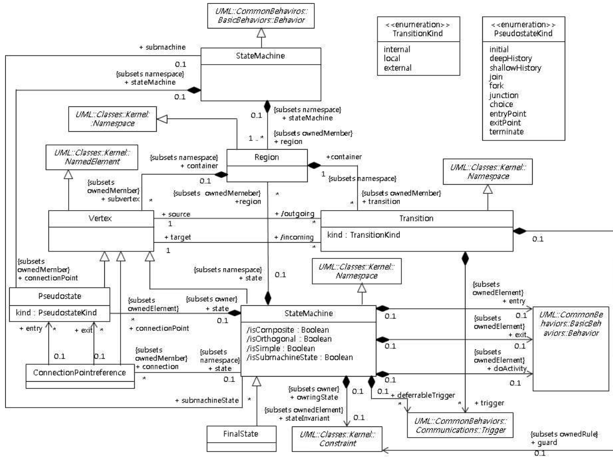
그림 3. UML 2.3에서 정의된 상태기계의 메타 모델[22] Fig. 3. Meta-model of UML 2.3 state machine diagram[22]
