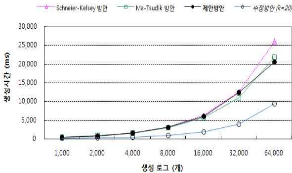
그림 2. 로깅 방안의 성능 비교 Fig. 2. Performance comparison of logging schemes
