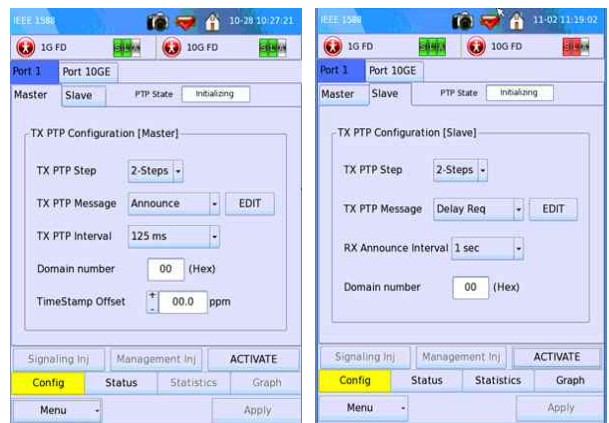
그림 4. TX PTP Configuration 화면 Fig. 4. TX PTP Configuration
