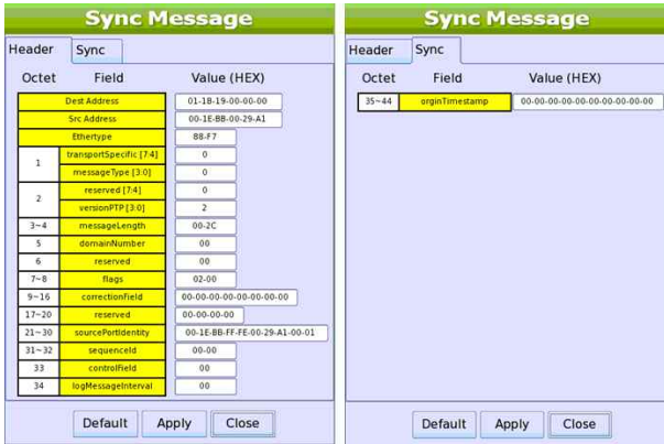
그림 5. TX PTP 메시지 편집 화면(Sync Message) Fig. 5. Edit screen of TX PTP message
