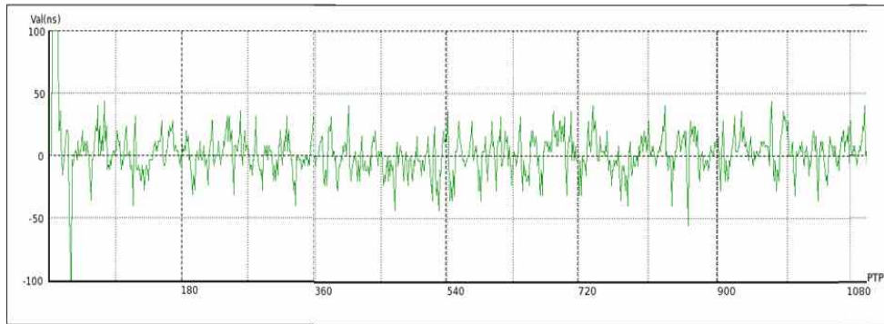
그림 9. Two-step일 때 Offset from Master 그래프 Fig. 9. Offset from Master of Two-step
