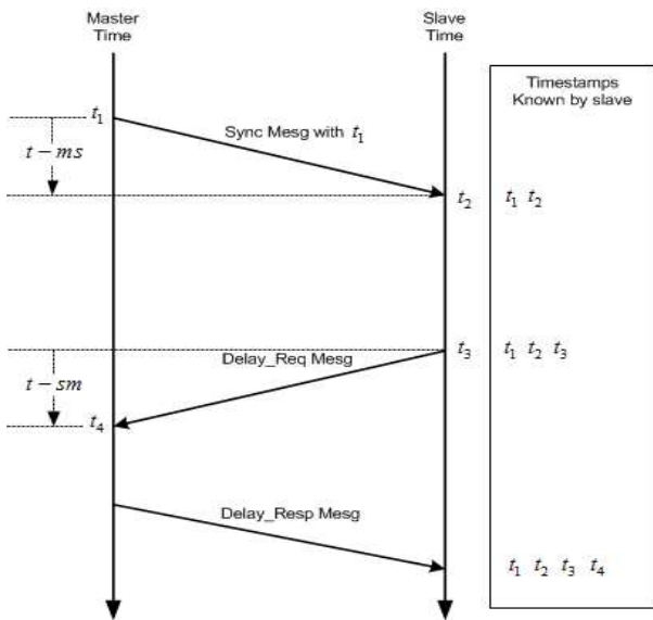
그림 2. One-step모드에서의 지연 요청-응답 메커니즘 Fig. 2. Delay request-response mechanism of One-step
