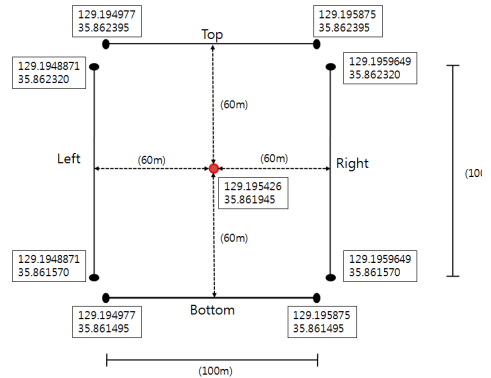
<그림 3> 구현된 프로그램의 정확성 검증 실험 데이터
