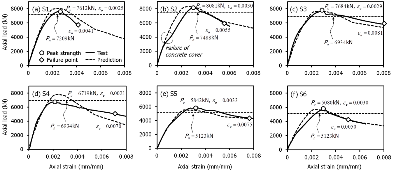
그림 6. 압축하중-변형률 관계
