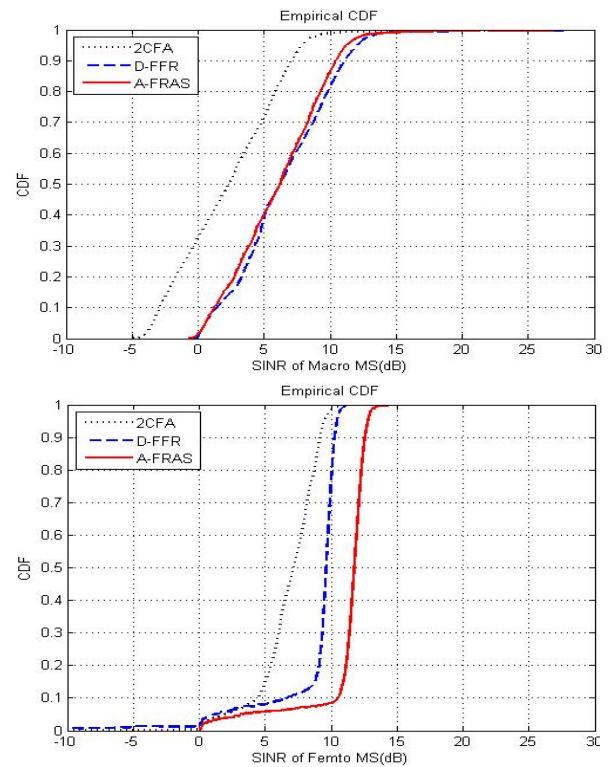
그림 12. 3 개의 알고리즘별 매크로 MS 와 펠토 MS 의 수신 SINR (펠토셀 = 100 개) Fig. 12. SINR distribution of Macro MS, Femto MS for three different algorithm (# of Femto BS = 100 EA)
