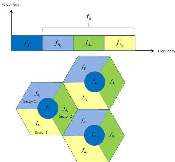
그림 1. FFR 기반의 매크로셀 주파수 할당 방식 Fig. 1. Frequency allocation scheme based FFR
