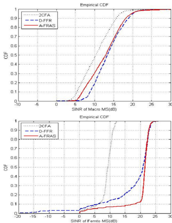
그림 8. 3 개의 알고리즘별 매크로 MS 와 펠토 MS 의 수신 SINR (펠토셀 = 20 개) Fig. 8. SINR distribution of Macro MS, Femto MS for three different algorithm (# of Femto BS = 20 EA)
