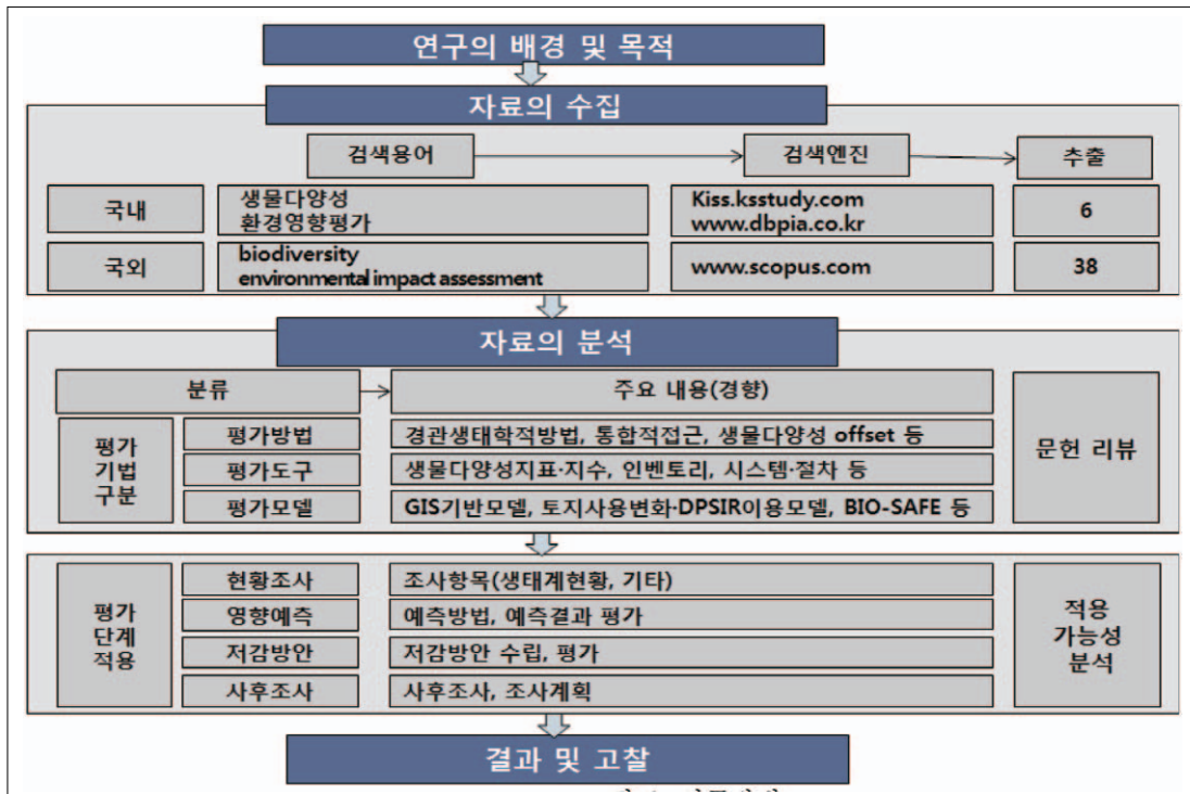
그림 1. 연구방법
