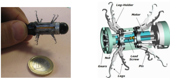
(a) 캡슐 외관 (a) CE shape (b) 캡슐 캐드 이미지 (b) CAD image of CE
