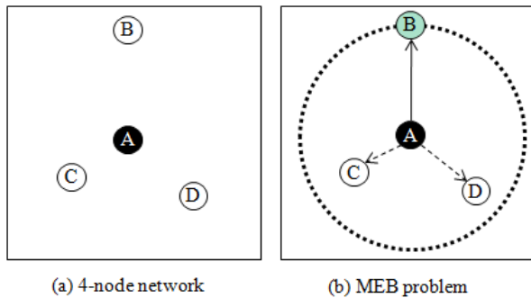
그림 1. 무선 네트워크의 MEB 문제 Fig. 1. MEB problem in wireless networks
