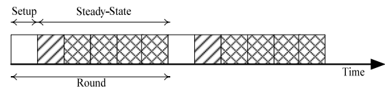
그림 1. LEACH 프로토콜 동작단계 Fig. 1. LEACH protocol phases
