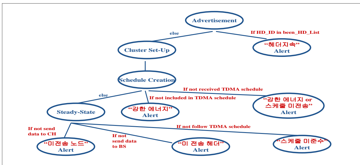
그림 5. 확장된 LEACH 프로토콜 상태 전이 다이어그램 Fig. 5. State Transition Diagram of Extended LEACH Protocol Specification
