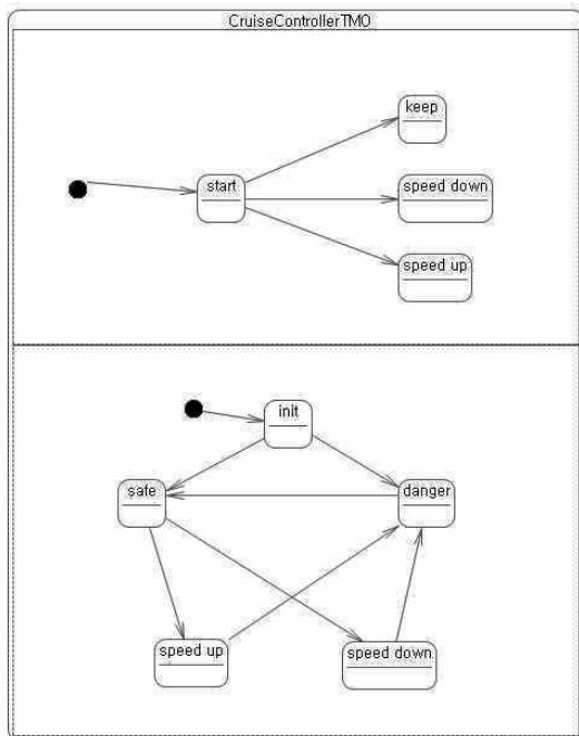
(그림 14) CruiseControllerTMO 클래스의 상태 머신 다이어그램
