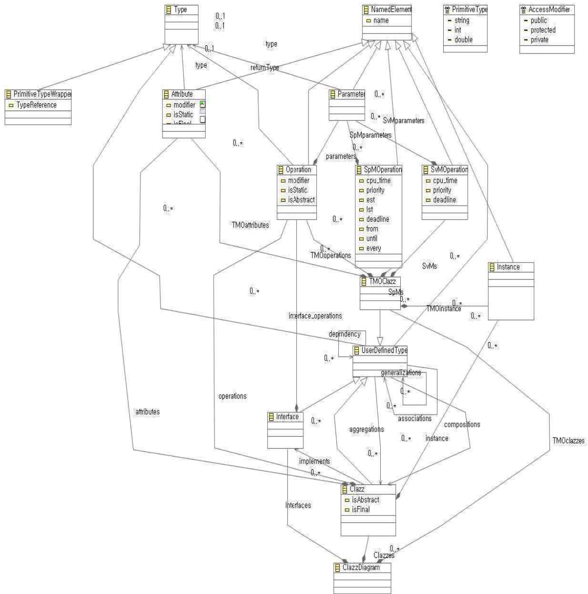
(그림 7) TMO 자원 확장된 클래스 다이어그램의 메타 모델
