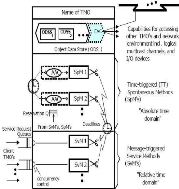
(그림 2) TMO 객체의 구조
