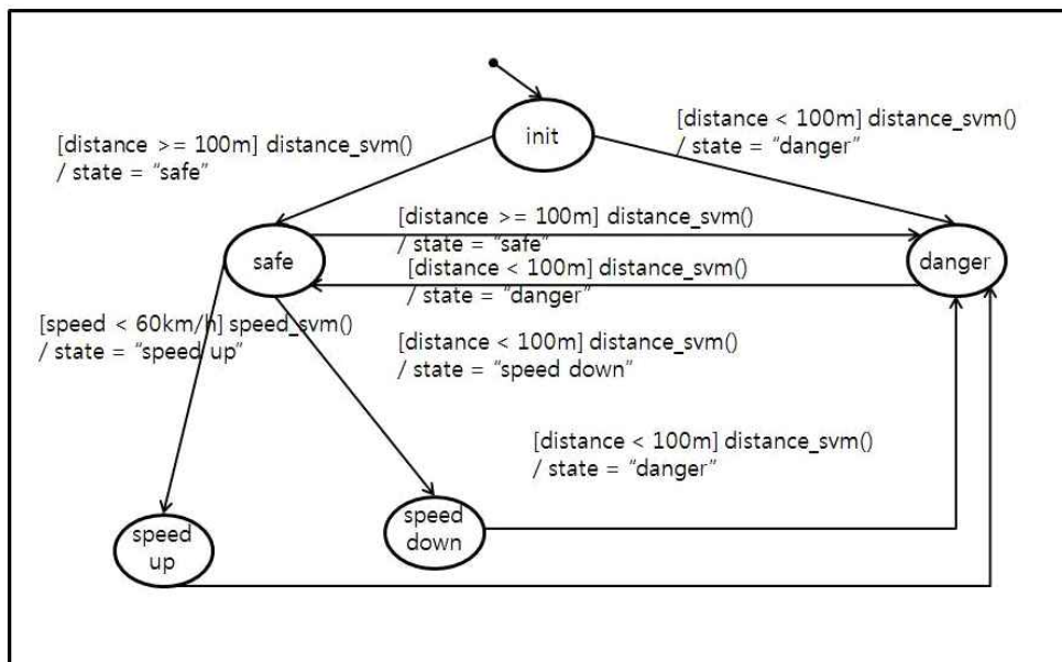
(그림 6) Control_SpM 메소드의 상태 머신 다이어그램
