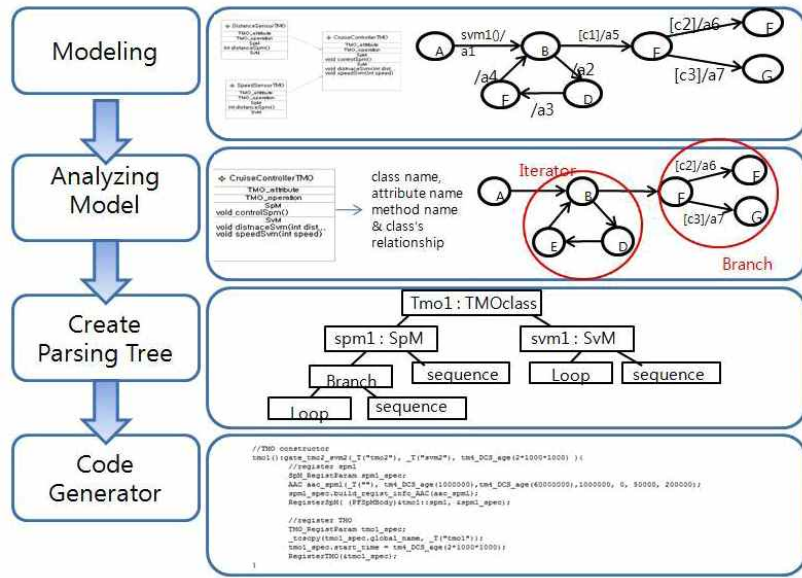
(그림 8) TMO 객체 모델 기반 코드생성 과정
