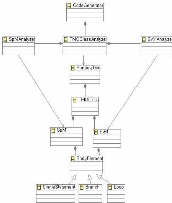
(그림 9) TMO 기반 코드 자동 생성기의 클래스 다이어그램
