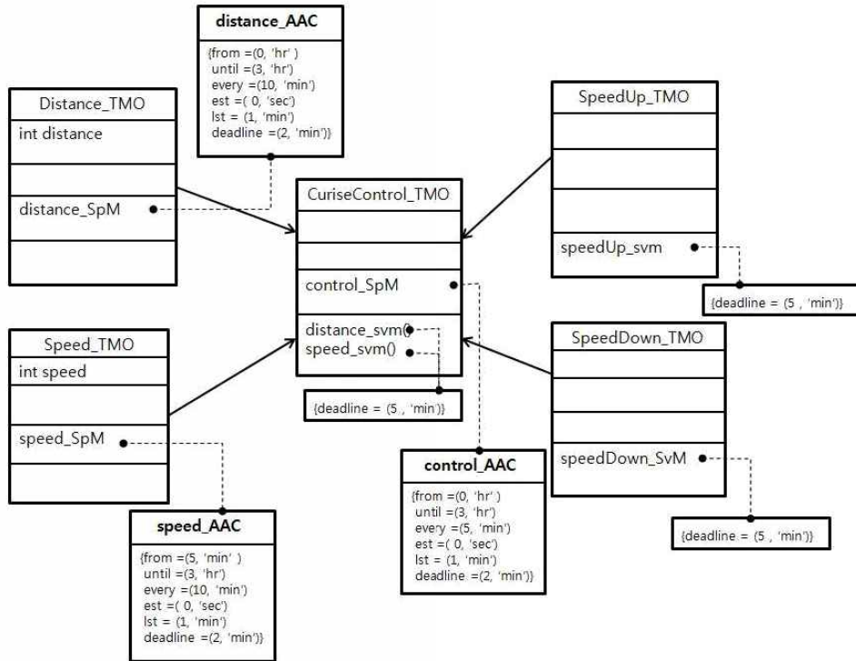
(그림 4) 순항 제어 시스템의 TMO 확장 클래스 다이어그램
