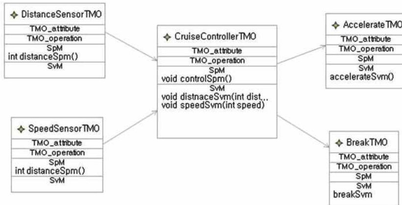
(그림 13) 순항제어 시스템의 클래스 다이어그램
