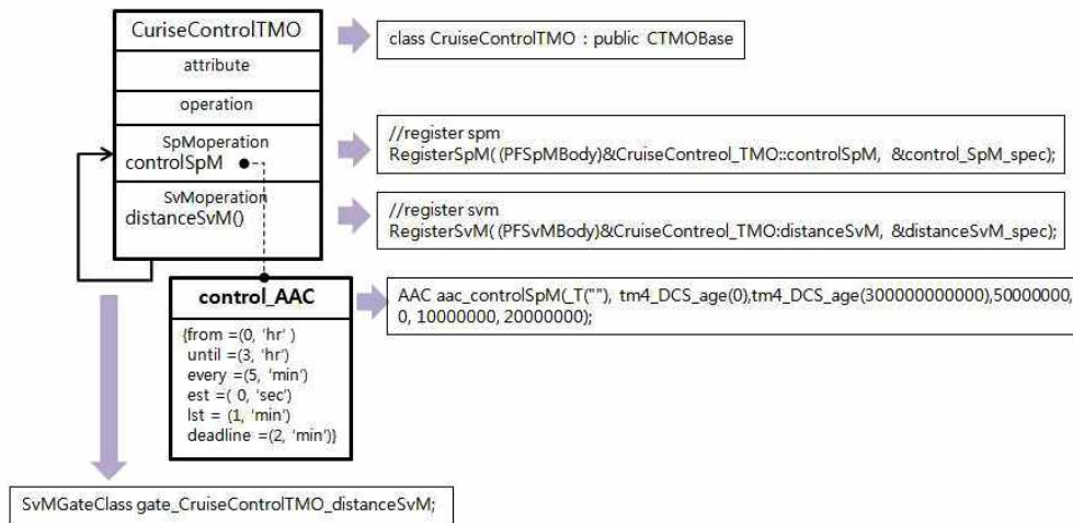
(그림 10) 클래스 다이어그램에서의 코드 생성 규칙
