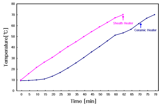
[그림 2] 스위스와 SiC계 발열체 승온 속도 비교 [Fig. 2] Rising curve of sheath and SiC heater
