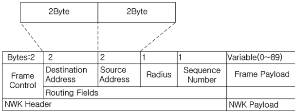
그림 4. 네트워크 계층의 프레임 형식 Fig. 4. The network layer frame format
