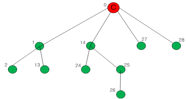
그림 3. C_m = 4, R_m = 2, L_m = 3 일 때의 주소 할당 Fig. 3. Address allocation when C_m = 4, R_m = 2, L_m = 3
