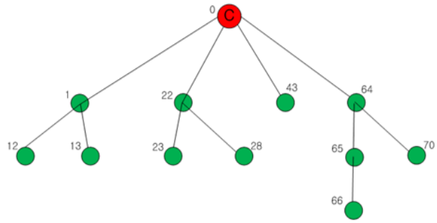
그림 2. C_m = R_m = 4, L_m = 3 일 때의 주소 할당 Fig. 2. Address allocation when C_m = R_m = 4, L_m = 3
