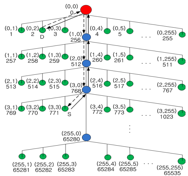
그림 6. (x, y) 좌표 평면에서의 라우팅 Fig. 6. (x, y) coordinates routing
