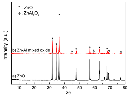
[그림 3] Al 첨가에 따른 XRD 분석 결과 [a] ZnO, b) Zn-Al mixed oxide]
