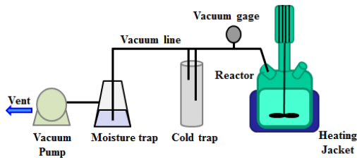
[그림 2] 합성장치의 개략도. [Fig. 2] Schematic diagram of the experimental apparatus for reaction
