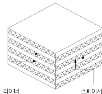
[그림 1] 전열교환 소자의 개략도
