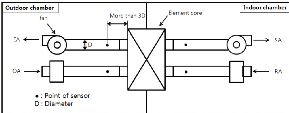
[그림 9] 전열교환기 성능 시험장치 개략도
