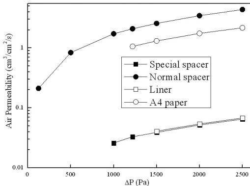
[그림 3] 각 스페이서 재질의 공기투과도
