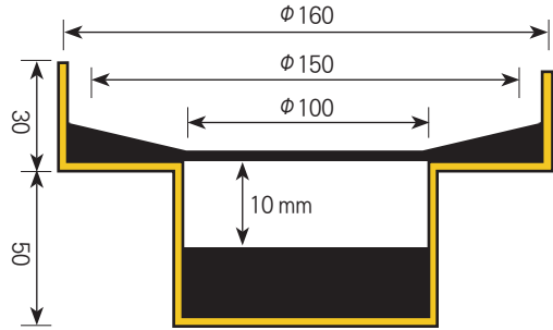
[그림 4] 투습성 측정용 투습컵
