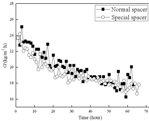
[그림 5] 각 시료별 투습량
