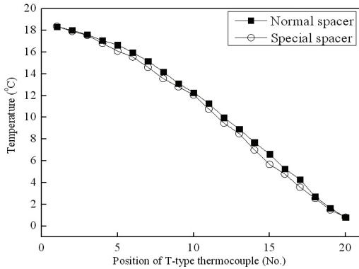
[그림 8] 각 스페이서 내부 온도분포 측정결과
