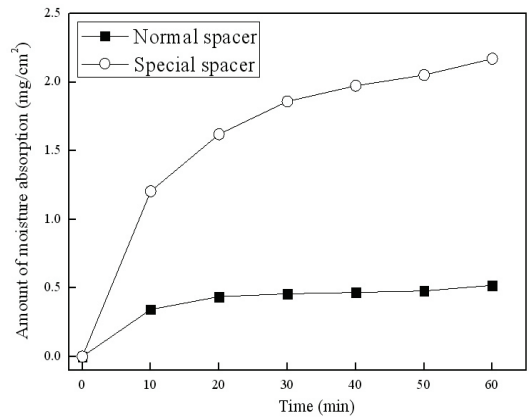
[그림 6] 각 시료의 흡습량
