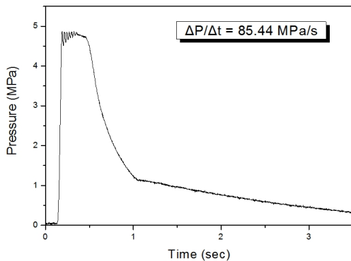
(c) 85.44 MPa/s
