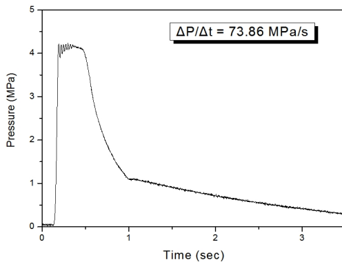
(b) 73.86 MPa/s
