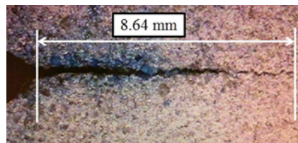
(c) 85.44 MPa/s
